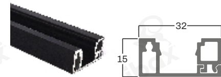
IPC 03 FOLDABLE (32 x 15 mm)
