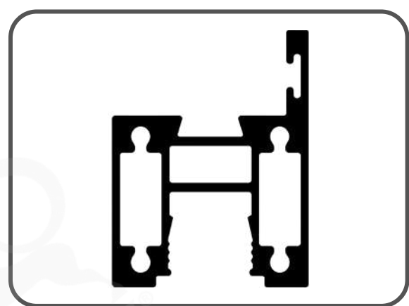
IPC-03 Door Jam 32x16
