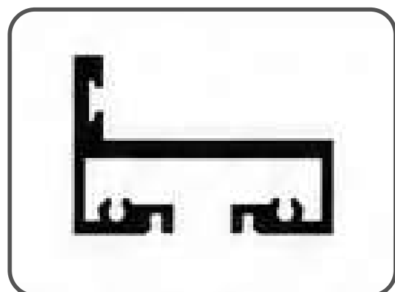
Door Jam 05 45x30
